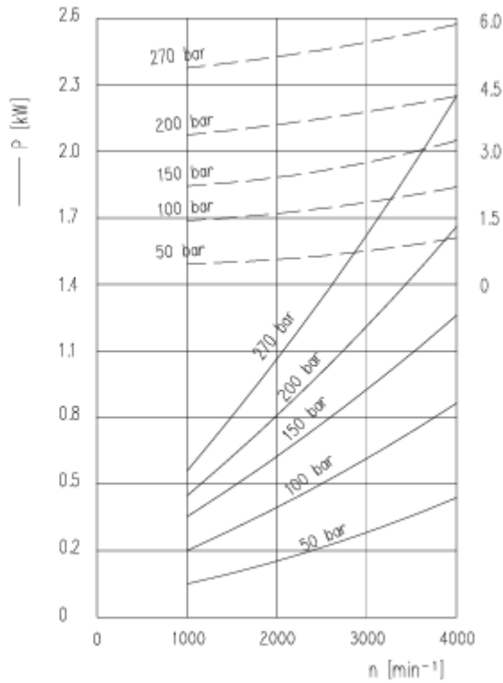
V=1.60CM3/r
