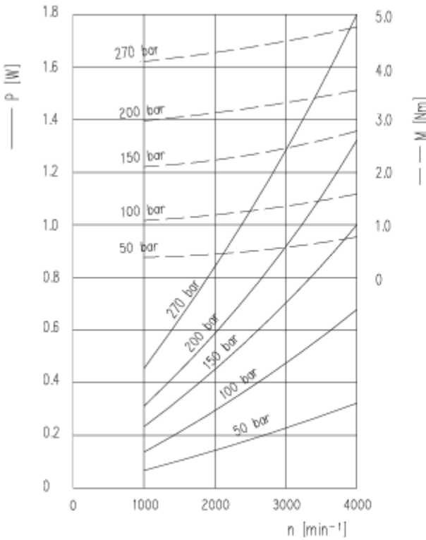
V=1.30CM3/r
